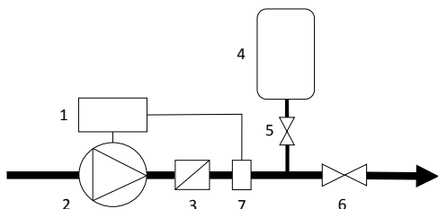
1: Wechselrichter; 2: Pumpe; 3: Rückschlagventil; 4: Ausdehnungsgefäß; 5: Absperrschieber; 6: Absperrschieber; 7: Drucksensor
